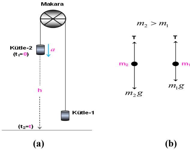
Şekil 5.1. Atwood aleti: (a): Düzenek, (b): Her bir kütleyle etki eden kuvvet
